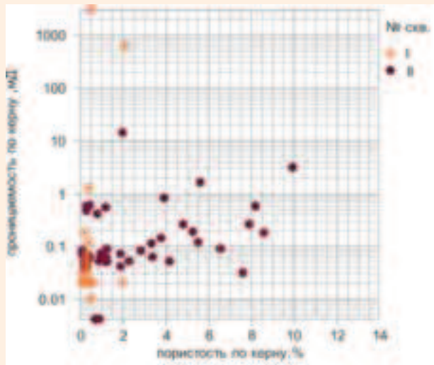
Рис. 3. Сопоставление пористости и проницаемости в отложениях доманикового типа. Св. I и II, Кашаевский участок
