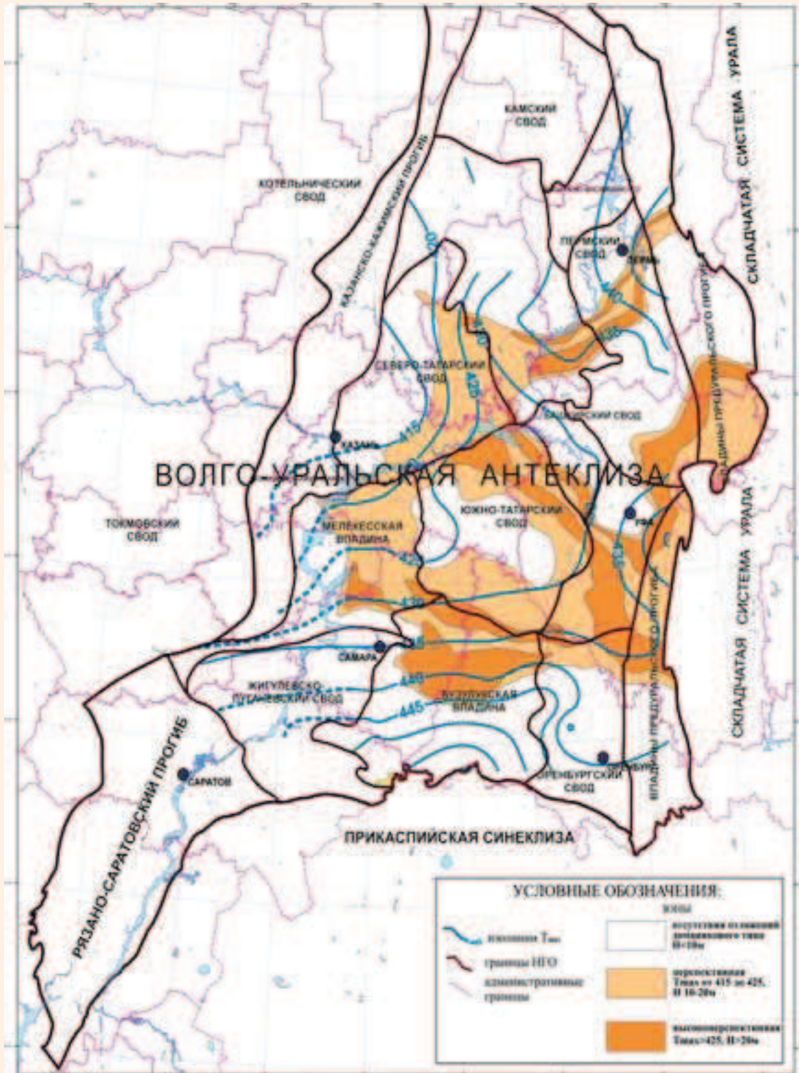
Рис. 5. Карта распространения перспективных зон отложений доманикового типа в евлановском и ливенском горизонтах Волго-Уральской НГО
